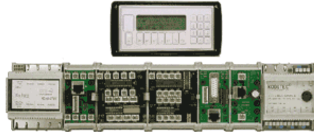
Système à microcontrôleur pour l'industrie, le contrôle de processus et la gestion de bâtiment KODITEC®
